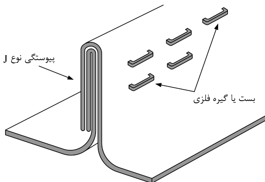
شکل ۵-۱۵- پیوستگی دو قطعه ژئوسنتتیک مجاور به وسیله بست‌های فلزی
