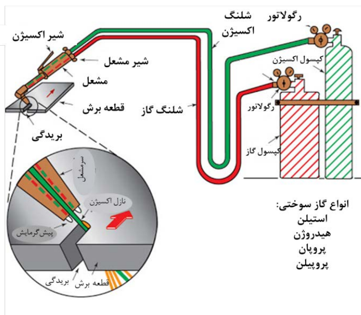
شکل ۴-۹- شماتیک تجهیزات یک فرایند برش داغ
