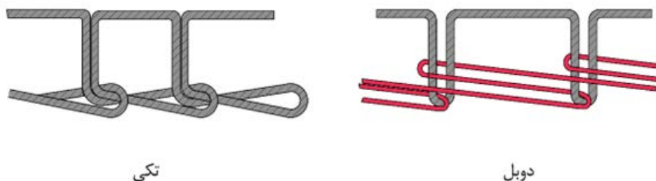
شکل ۵-۱۲- دو نوع کوک‌زنی (تکی و دوبل)
