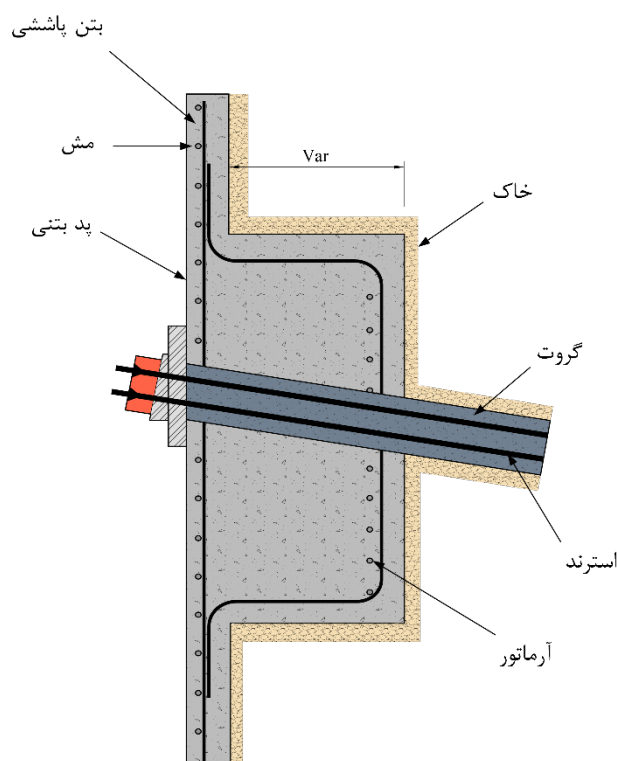
شکل ۵-۵- پد بتنی
