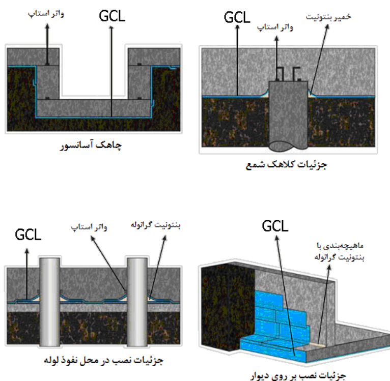
شکل ۵-۲۷- نحوه اجرای ژئوکمپوزیت رسی در اطراف سرشمع و دیواره گود و محل اتصال
