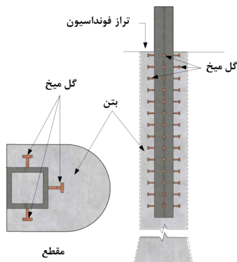
شکل ۵-۷- نحوه اتصال ستون فلزی به شمع بتنی
