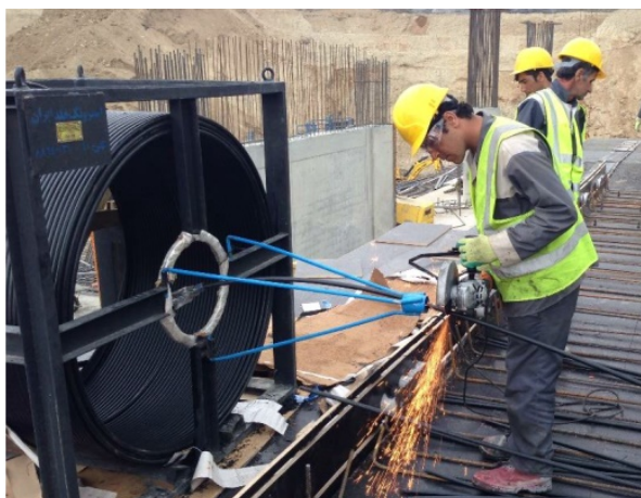
پ) قرقه تاندون‌ها و باز کردن تاندون‌ها و جایگذاری آن‌ها توسط ابزار هدایت از روی قرقه (انتهای مرده تاندون در فاصله ۵۰ میلی‌متری قالب جداره قرار می‌گیرد)
