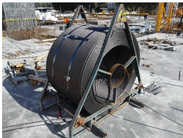
پ) قرقه تاندون‌ها و باز کردن تاندون‌ها و جایگذاری آن‌ها توسط ابزار هدایت از روی قرقه (انتهای مرده تاندون در فاصله ۵۰ میلی‌متری قالب جداره قرار می‌گیرد)
