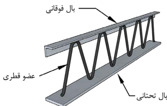
شکل ۴-۲۱- اجزای تیرچه فولادی با جان باز
