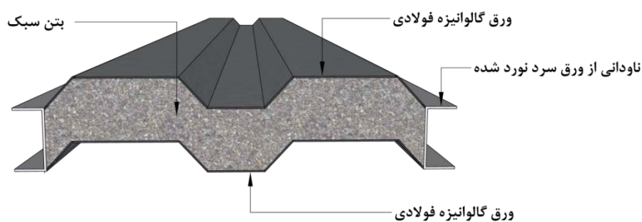
شکل ۶-۲۳- دال مرکب فولادی و بتنی
