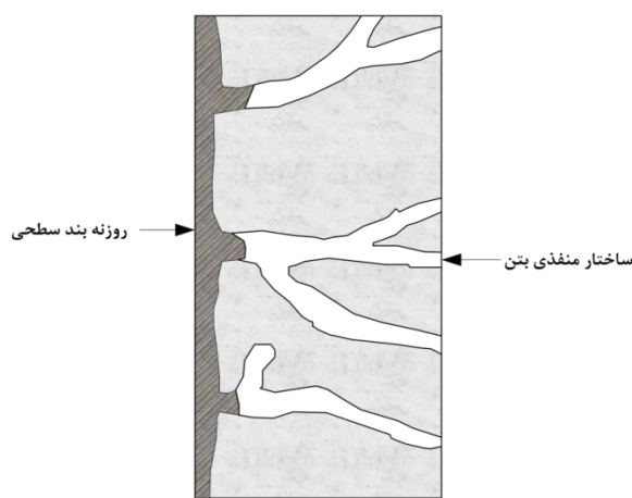
شکل ۶-۲۶- نمایشی از رخنه‌بند سطحی
