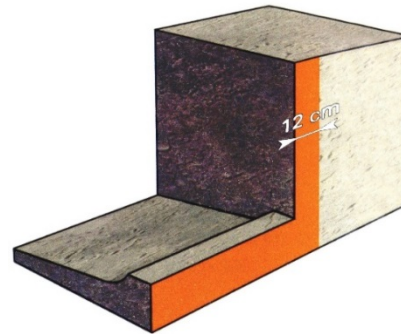
شکل ۱۲-۲۹- مثال آماده‌سازی سطوح بتنی محل نصب پنجره و در با تکیه‌گاه همباد
