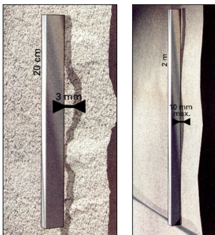
شکل ۱۲-۲۸- رواداری مجاز صاف بودن کلی و موضعی
