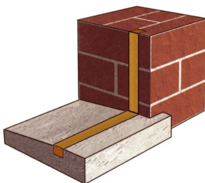
شکل ۱۲-۴۰- کاربرد پیش قاب چوبی در روش نصب توکار
