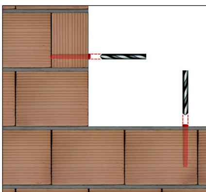
شکل ۱۲-۴۸ جزئیات اجرایی آماده‌سازی اتصال قاب در و پنجره، در صورت اجرای بلوک‌های کناری با حفره‌های قائم
