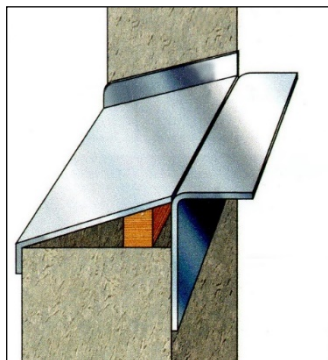
شیب حداقل ۱۰ درصد برای زیرپنجره آلومینیومی
