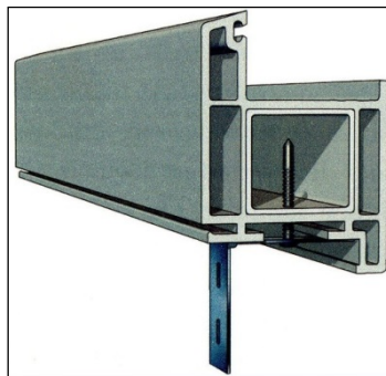
شکل ۱۲-۵۱- اتصال نبشی به قاب با پیچ سر مته‌ای
