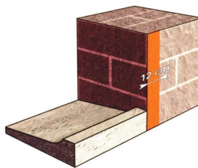
شکل ۱۲-۳۳- آماده‌سازی سطوح یک گشودگی ساخته‌شده از بلوک یا آجر سوراخ‌دار با تکیه‌گاه پیش‌ساخته در حالت نصب روکار
