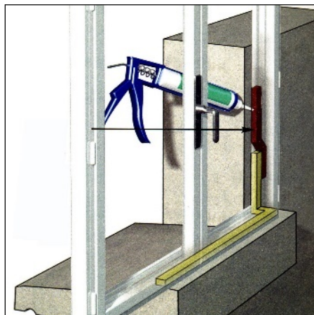
شکل ۱۲-۵۸- همپوشانی بتانه با اسفتج در درزبندی
