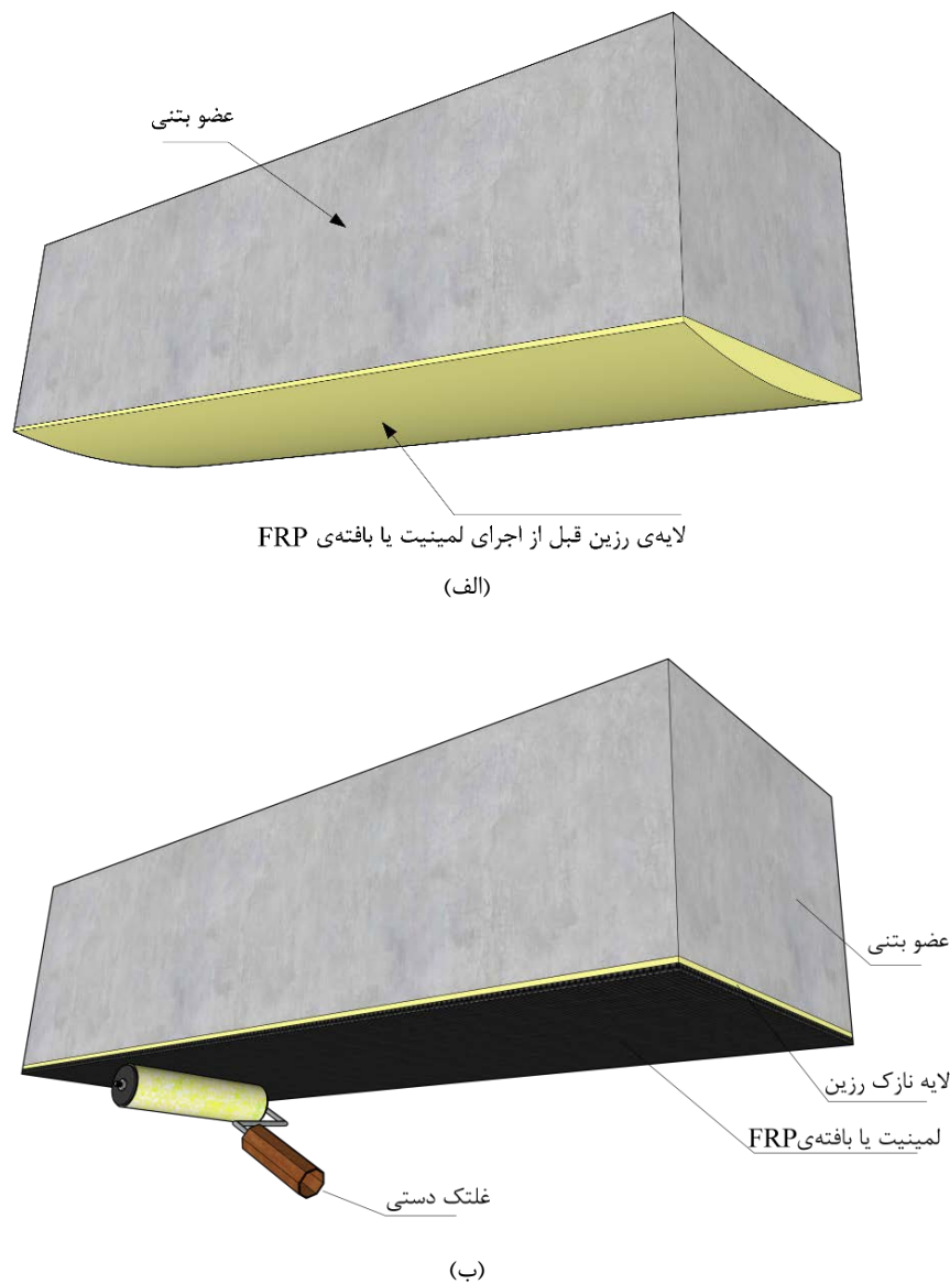
شکل ۱۴-۴۴ الف) آغشته کردن عضو بتنی با لایه‌ی نازک از رزین زیر لمینیت و یا بافته‌ی FRP؛ ب) کشیدن غلطک (کاردک) مناسب روی سطح نوار یا ورق FRP جهت از بین بردن حباب هوا
