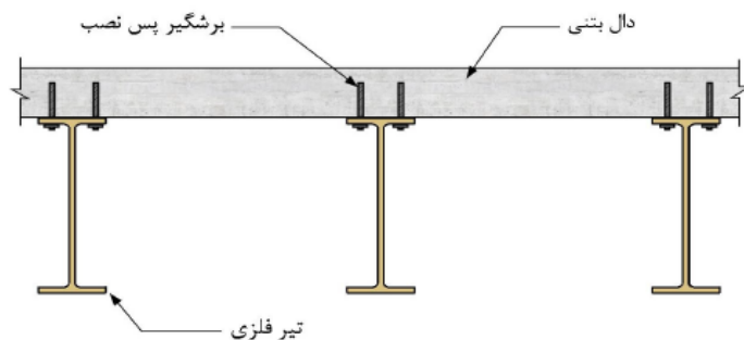
شکل ۱۴-۷۸- برشگیر پس نصب
