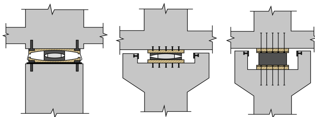
الف- جداساز لاستیکی با هسته سربی ب- جداساز اصطكاكي تك پاندولی پ- جداساز اصطكاكي سه پاندولی شکل ۱۴-۱۵۳- جزئیات نصب ایمن انواع مختلف جداسازها در بالای ستون با پایه‌های اطمینان یا رینگ محافظ پیرامونی
