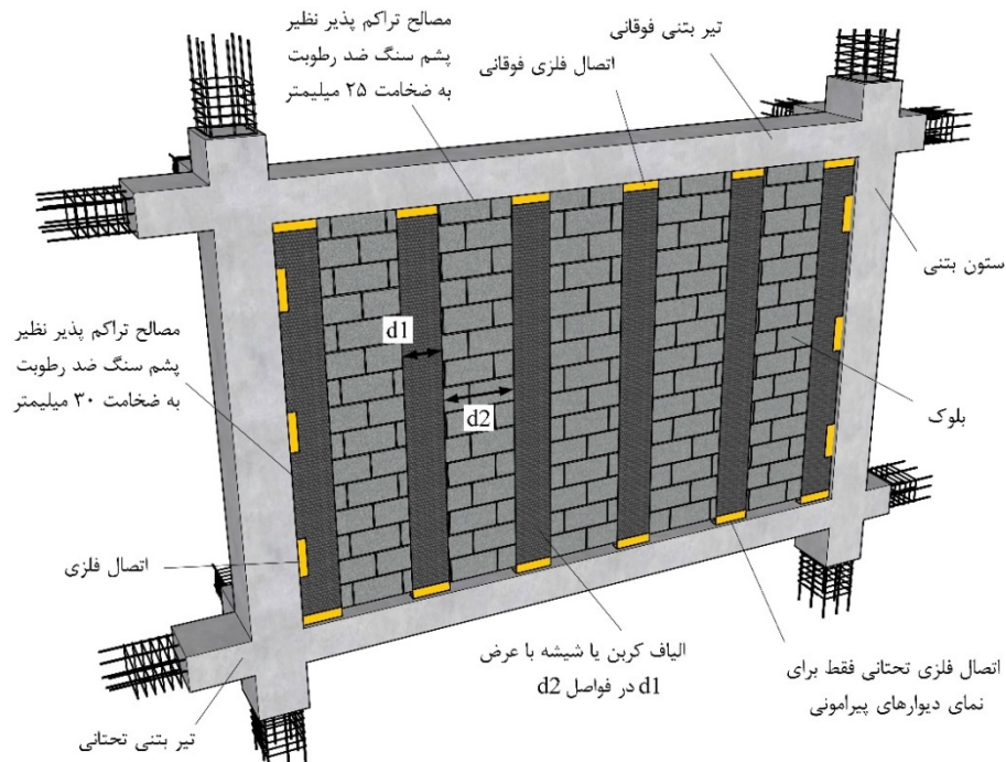
شکل ۱۴-۱۸۱- بهسازی لرزه‌ای دیوارها با استفاده از نوارهای شبکه الیاف
