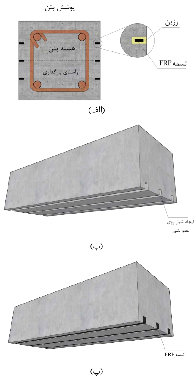
شکل ۱۴-۴۵- روش نصب در نزدیک سطح (NSM)؛ (الف) نحوه تقویت ستون به صورت شماتیک؛ (ب) ایجاد شیار در راستای مورد نظر روی عضو بتنی؛ (پ) قرار دادن تسمه (نوار) داخل شیار و تزریق رزین به صورت همزمان
