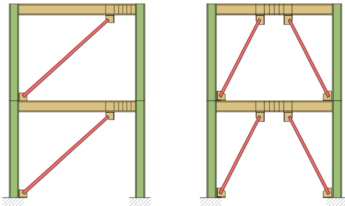
شکل ۹۸-۱۴- مهاربند واگرای فولادی
