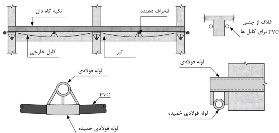
شکل ۱۴-۵۶- انحراف‌دهنده مسیر
