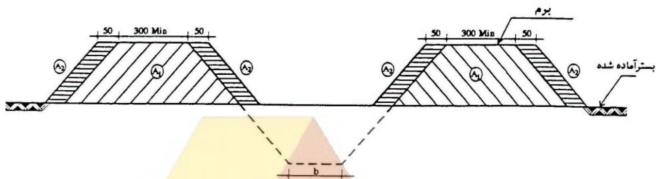
شکل ۳-۴. شمای مقطع خاکریزی
