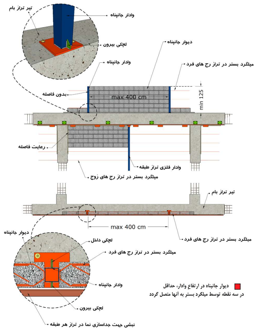
شکل ۱۲-۳۳- مهار جان پناه بنائی توسط وادی فلزی
