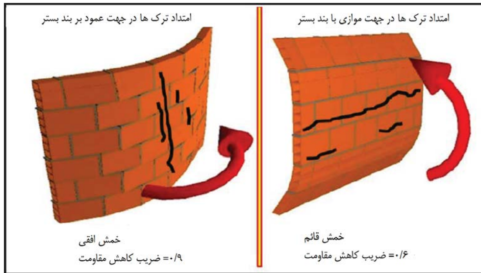
شکل ۳-۱۲- خمش افقی و قائم به همراه ضرایب کاهش مقاومت خمشی در دیوار بنایی دارای میلگرد بستر افقی
