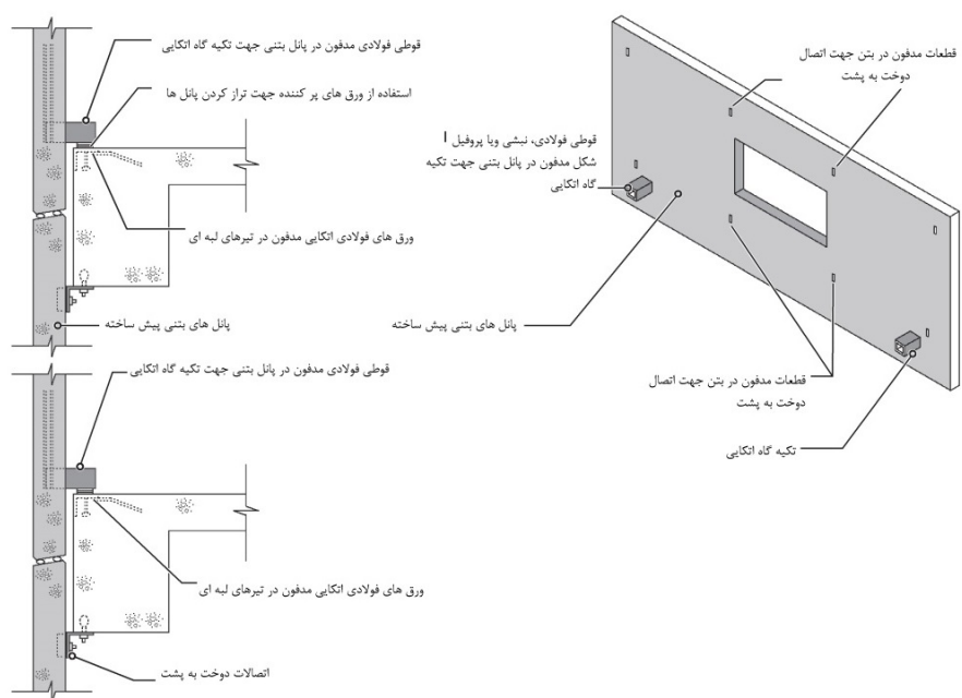
شکل ۱۰-۴- تیپ اتصالات تکیه‌گاهی یک پانل بتنی پیش ساخته
