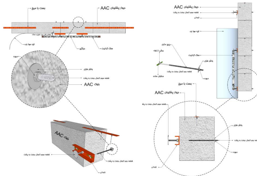
شکل ۴-۱۸ - نمونه‌ای از جزئیات اجرای نمای سنگی خشک بر روی دیوار عایق و مهار آن به دیوار پستی
