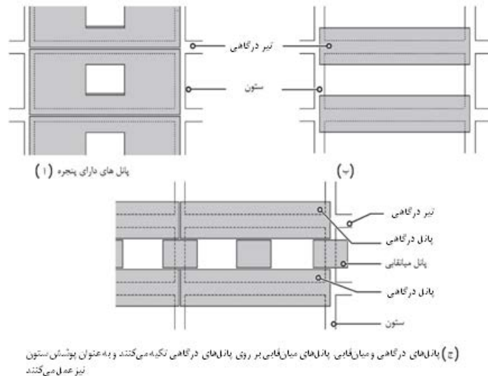
شکل ۱۰-۳- نمونه‌هایی از انواع اشکال پانل‌های بتنی پیش‌ساخته
