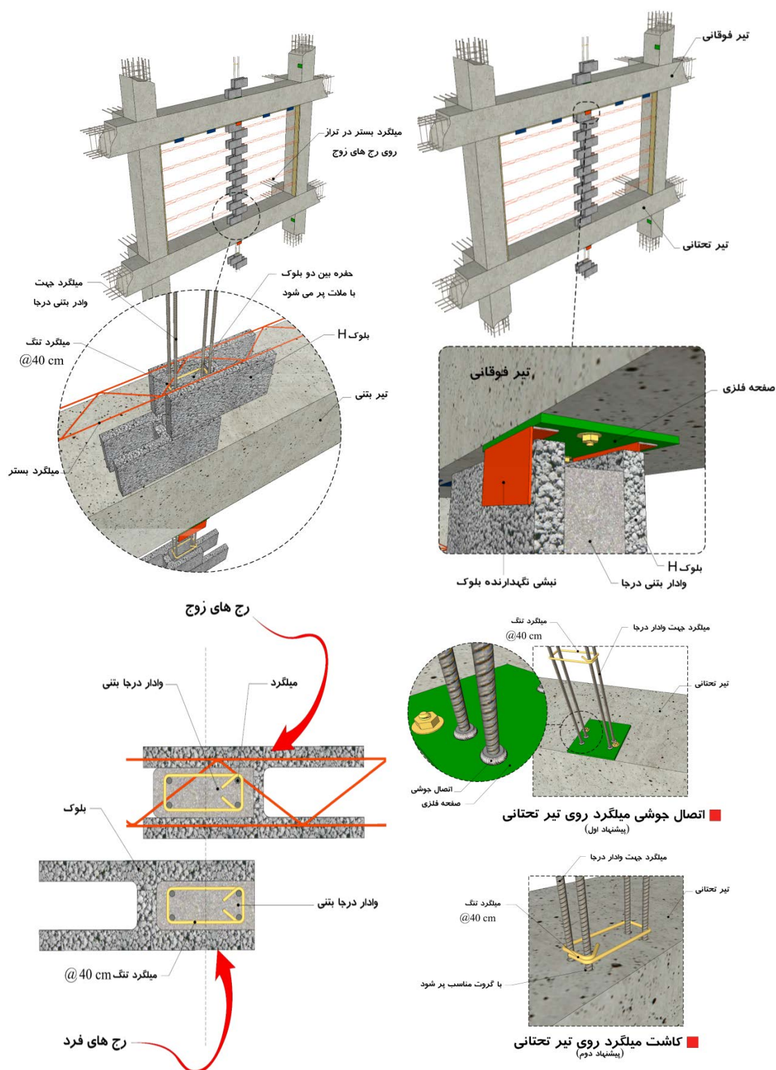
شکل ۱۲-۸- نمونه‌ای از وادار بتنی و جزییات اجرایی آن در دیوار بلوکی
