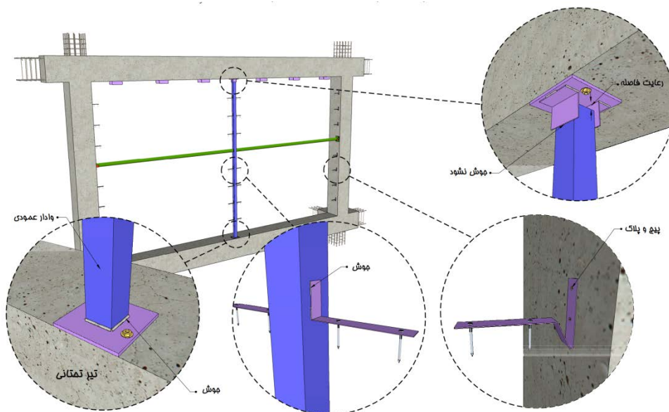
شکل ۱۲-۱۱- جزییات اجرایی اتصال تیرک و وادار در دیوار با ارتفاع بیش از ۳/۵ متر
