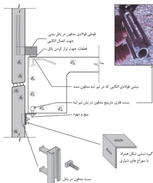
شکل ۷-۱۰- نمونه‌ای از اتصال دوخت به پشت
