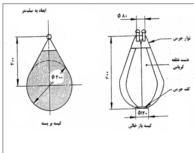
شکل ۳-۲- کیسه کروی مخروطی پنجاه کیلوگرمی
