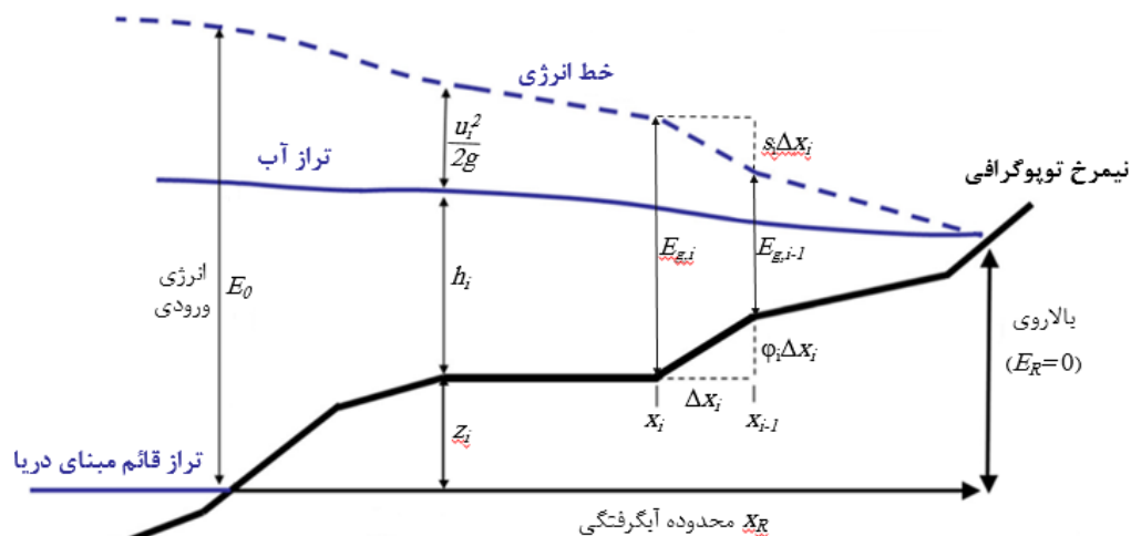
شکل ۲-۱: کمیت‌های مربوطه در روش تحلیل شیب خط انرژی
