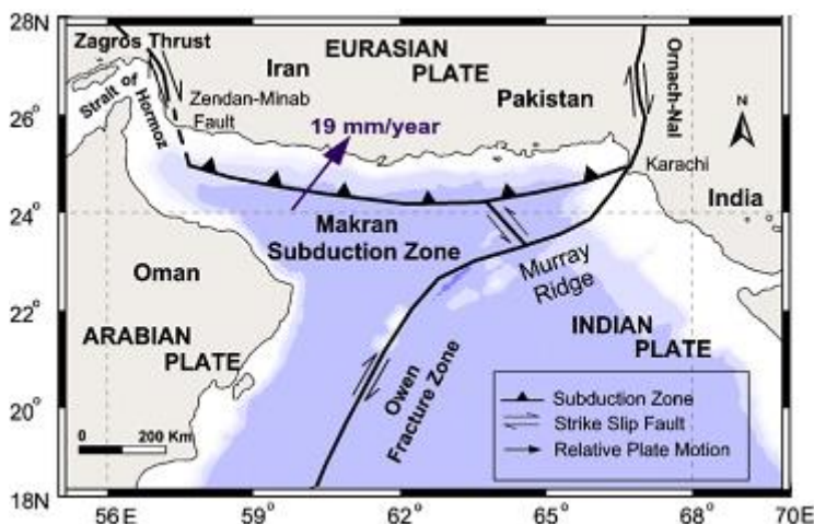
شکل ۷-۱: موقعیت ناحیه فروانش مکران در شمال غرب اقیانوس هند (Heidarzadeh و همکاران، ۲۰۰۸)
