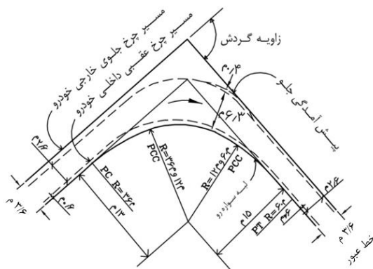
قوس مرکب سه مرکزی با شعاع‌های ۱۲ متر - ۳۶ متر - ۶۰ متر و عقب نشینی ۳۱ متر
