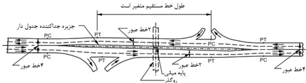
تعریف متقارن حول محور مرکزی - A -
