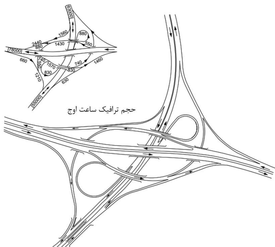
شکل ۳۶-۶- تبادول جهتی با دو اتصال نیمه جهتی
