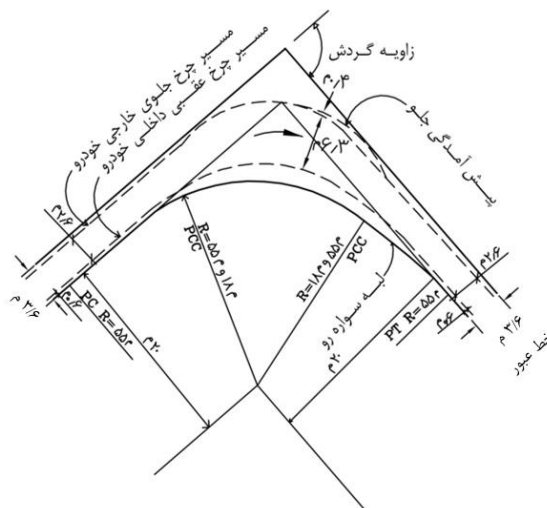
قوس مرکب سه مرکزی با شعاع‌های ۱۸ متر - ۵۵ متر - ۵۵ متر و عقب نشینی ۲ متر
