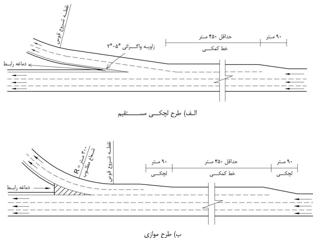
شکل ۶-۷- حالت‌های متداول رابط خروجی دو خطه
