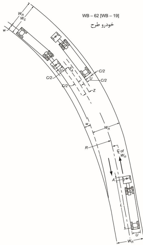
شکل ۵-۵- تعریف راه در قوس افقی
