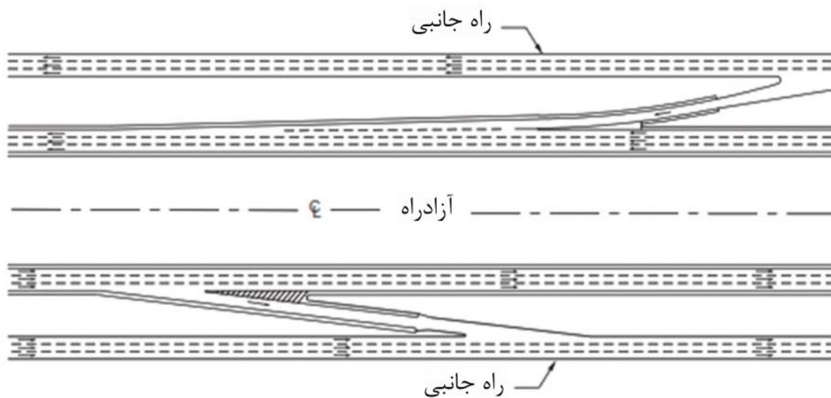
شکل ۶-۱۳- راه جانبی سه خطه در دو سمت آزادراه و رابط‌های کناری
