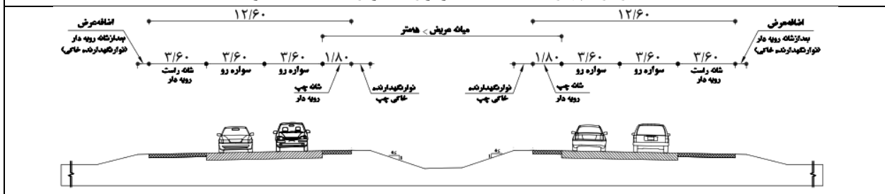
F10 - آزادراه چهار خطه با DDHV برابر و بیشتر از ۲۵۰ با میانگانه عریض
