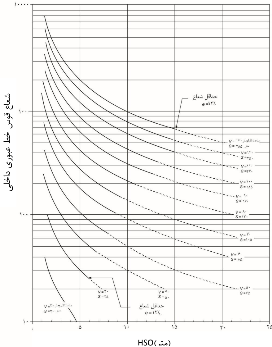
شکل ۵-۸- تعیین HSO در قوس افقی برای فاصله دید توقف فاصله خط دید افقی (مرکز خط داخل تا مانع) (متر)
