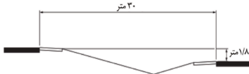
(ب) - فرونشسته با خط پروژه‌های مستقل
