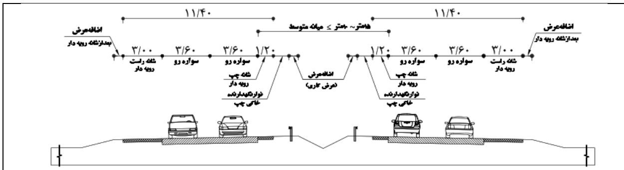
F7 - آزادراه چهار خطه با DDHV کمتر از ۲۵۰ با میانگانه متوسط
