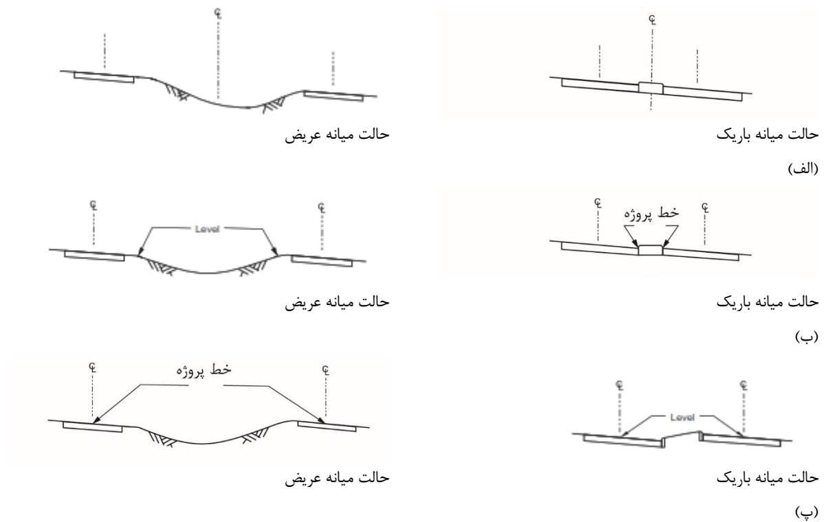
شکل ۵-۴- اعمال بریلندی در راه‌های مجزا
