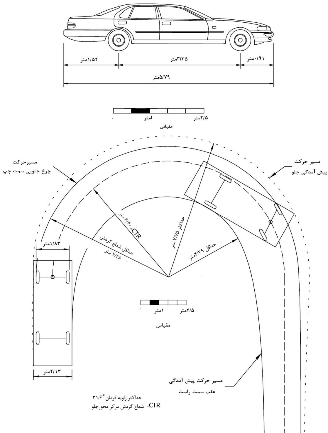
شکل ۲-۴- حدافل مسیر گردش برای وسیله طرح سواری
