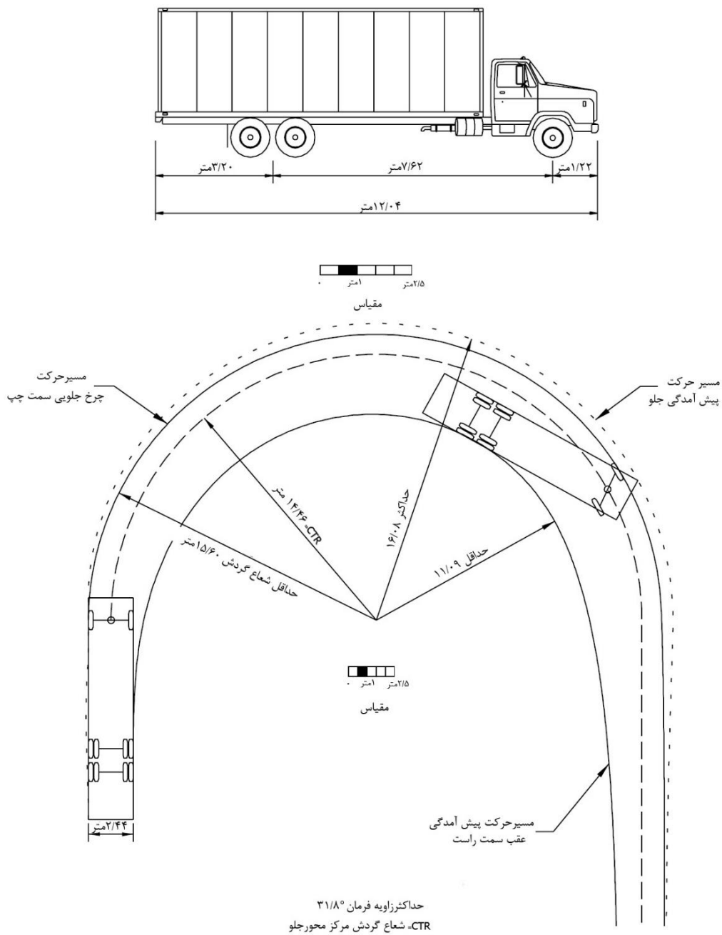
شکل ۴-۴- حدافل مسیر گردش برای وسیله طرح کامیون نوع ۲
