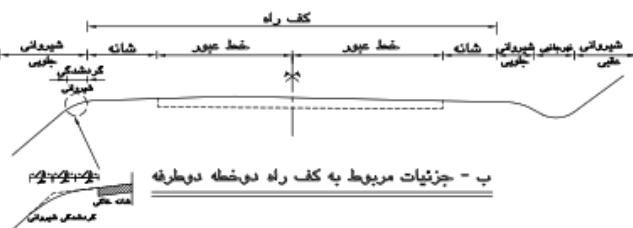
شکل ۶-۲- اجزای مقطع عرضی در راه‌های دو خطه و چهار خطه
