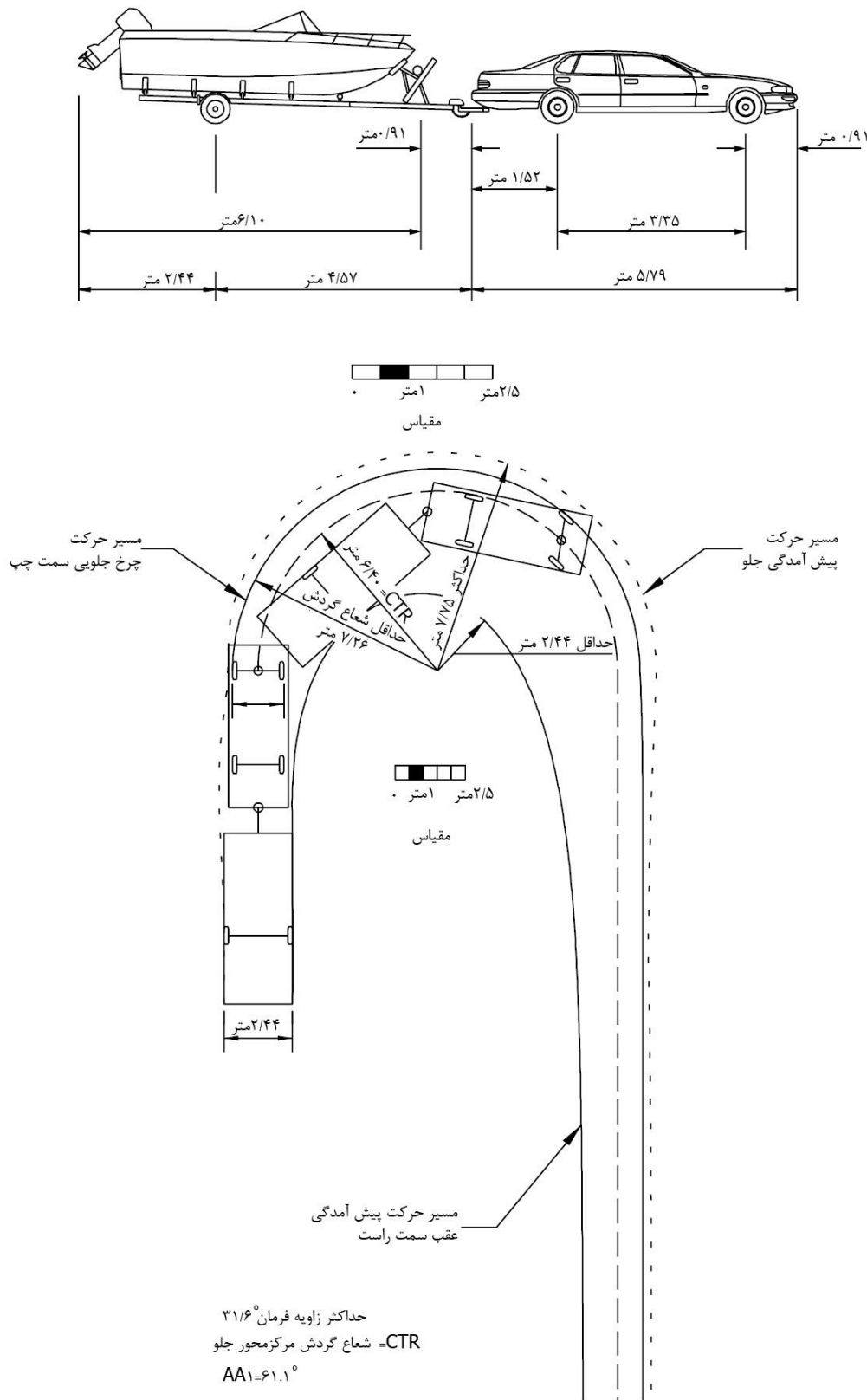
شکل ۴-۱۰- حدافل مسیر گردشی برای وسیله طرح سواری با یدک قایق
