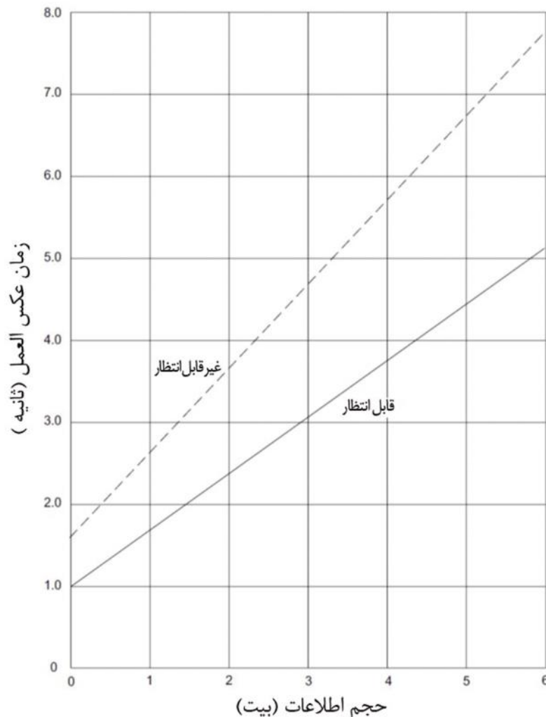
شکل ۴-۱- هشتماد و پنجمین صدک زمان عکس العمل رانندگان با توجه به اطلاعات دریافتی قابل انتظار و غیرقابل انتظار
