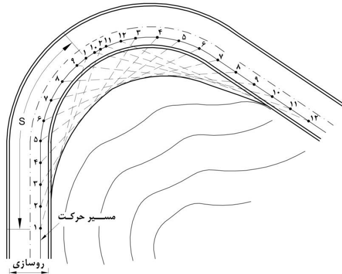
شکل ۷-۵ - نحوه تعیین میزان بی‌مانع نمودن محوطه در قوس افقی
