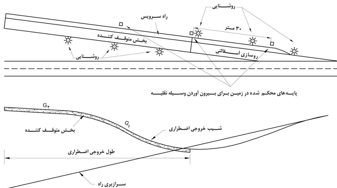
شکل ۵-۲۰- نمونه رمپ فرار اضطراری
