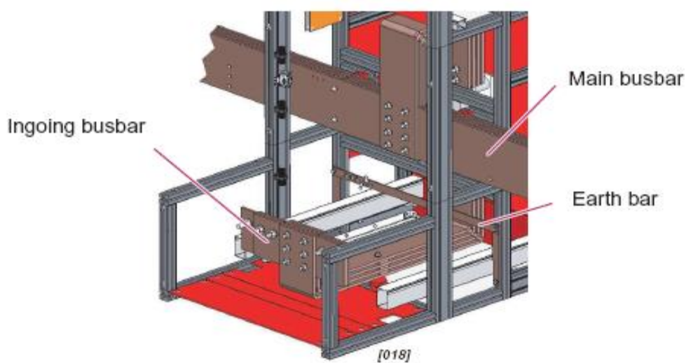
شکل ۳-۴ نمای باسبار پشت
