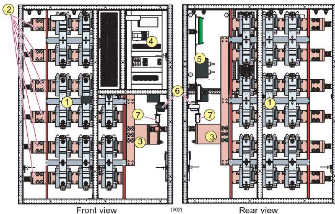
شکل ۴-۸ نمای جلو تابلو یکسوساز کثش
