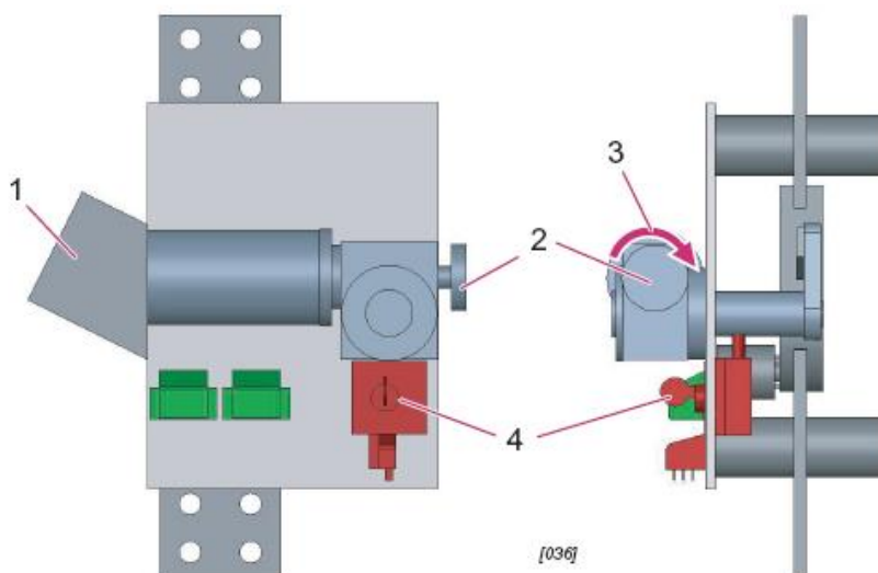
شکل ۴-۶۵ عملکرد MRID2
