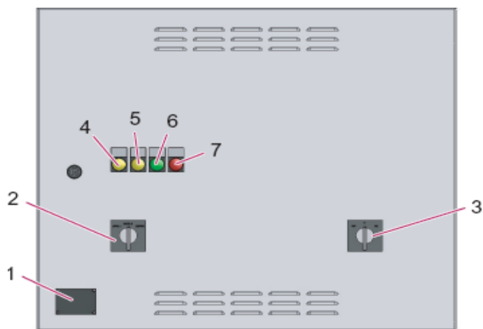
شکل ۳-۲۲ نمای درب محفظه کنترل
