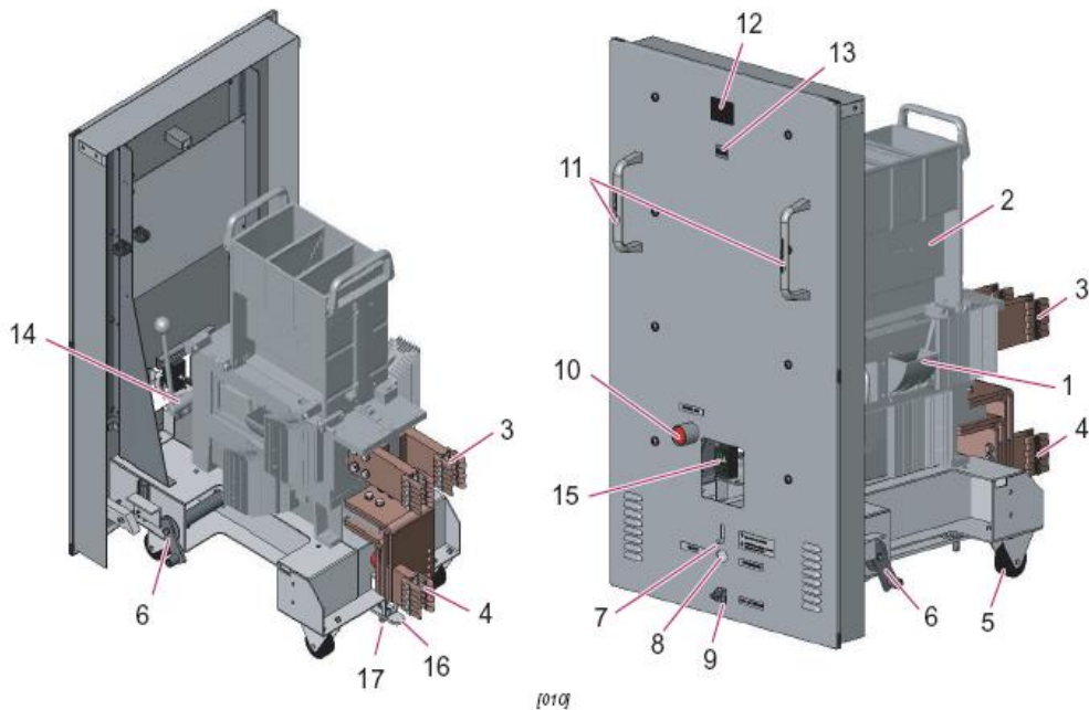
شکل ۴-۲۳ ارابه کشویی کلید HSCB
