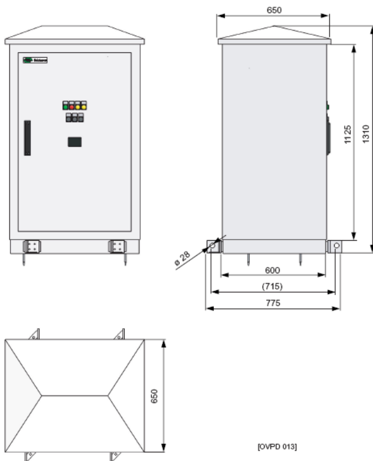
شکل ۴-۵ ابعاد عرض و ارتفاع تابلو ND20
