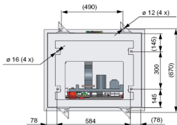
شکل ۴-۵ ابعاد تابلو ND20
