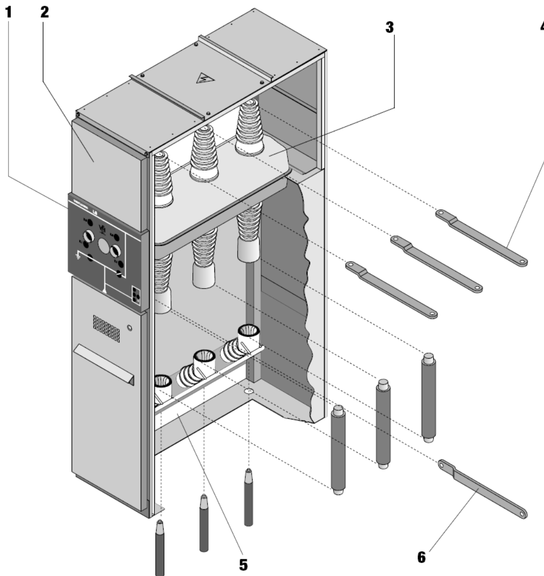
شکل ۸- اجزای یک تابلو UNIFLOURC
