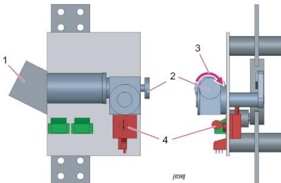
شکل ۴-۶۴ عملکرد MRID1
