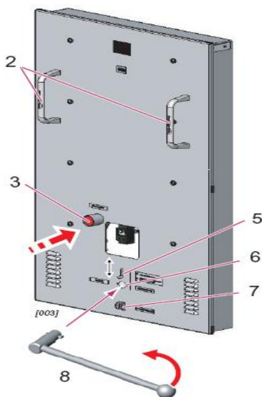
شکل ۴-۲۴ نمای جلوی ارابه کشویی
