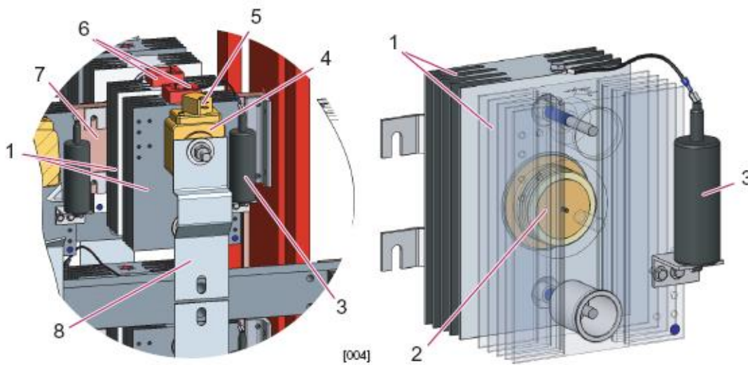
شکل ۴-۱۱ بلوک دیود
