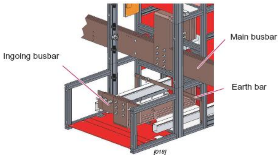
شکل ۴-۳۸ نمای باسپار پشت
