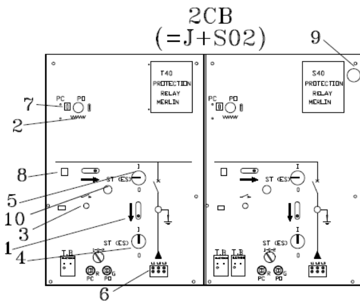
شکل ۴-۷۳ تجهیزات تابلو 2CB
