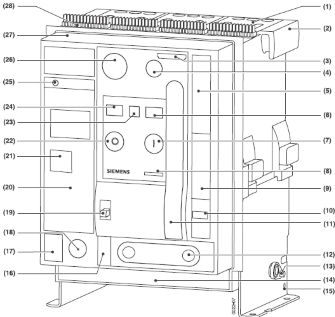
شکل ۲۵ - اجزای ACB
