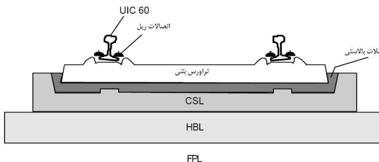
شکل ۲-۸ خط بدون بالاست طرح‌های کمپ
