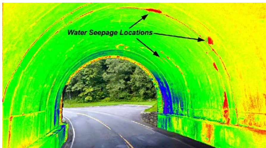
شکل ۱-۱۹ به کارگیری دمانگاری مادون قرمز در بازرسی تونل
