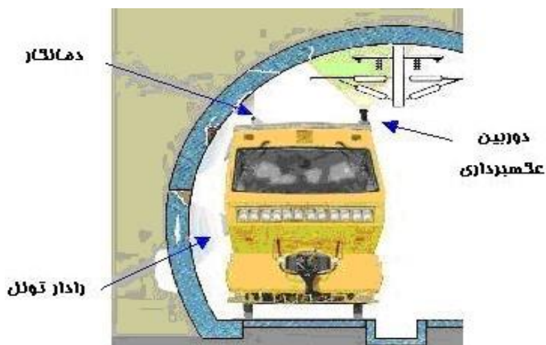
شکل ۳۵ → تجهیزات قطار بازرسی
