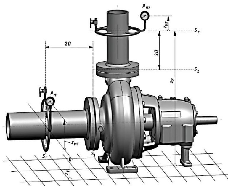
شکل الف-۱ نمایش ایزومتری تعیین ارتفاع کل پمپ
