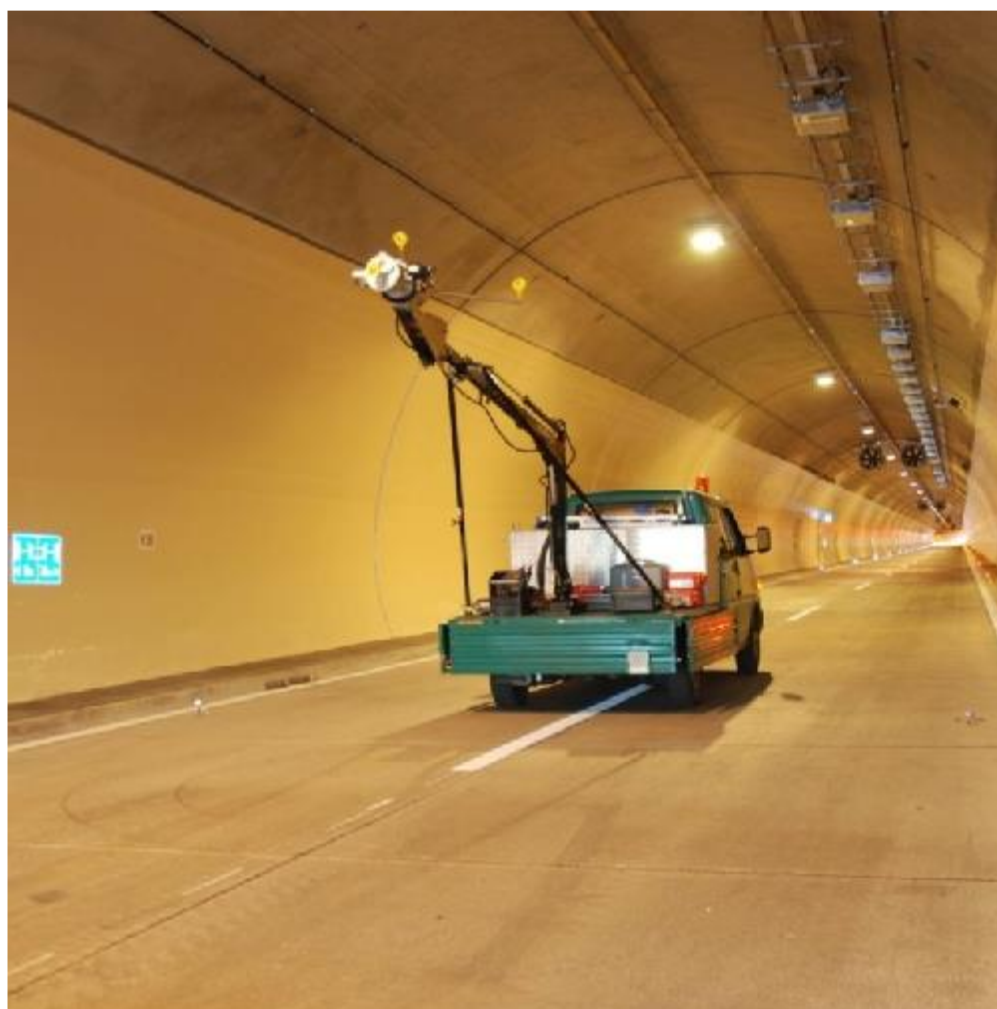
شکل ۸-۱ استفاده از دوربین برای بازرسی چشمی
