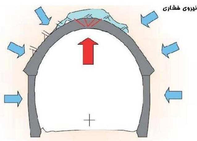
شکل ۱-۲۷ ایجاد ترک‌های کششی به دلیل توزیع غیریکنواخت نیروی فشار بر روی پوشش تونل
