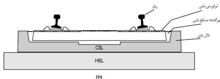
شکل ۲-۵ خط بدون بالاست طرح رهدا سنبرگ
