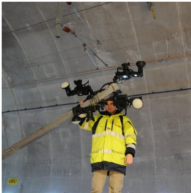
شکل ۳۲- ماشین عکسبرداری
