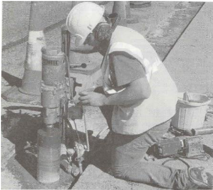
شکل ۵-۴ تنظیمات کلی آزمایش مغزه‌گیری از بتن
