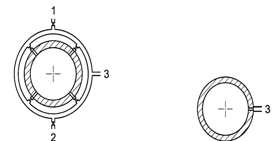
الف) رتبه ۱: ۴ انشعاب فشار که توسط یک حلقه چند راهه به هم متصل شده‌اند
