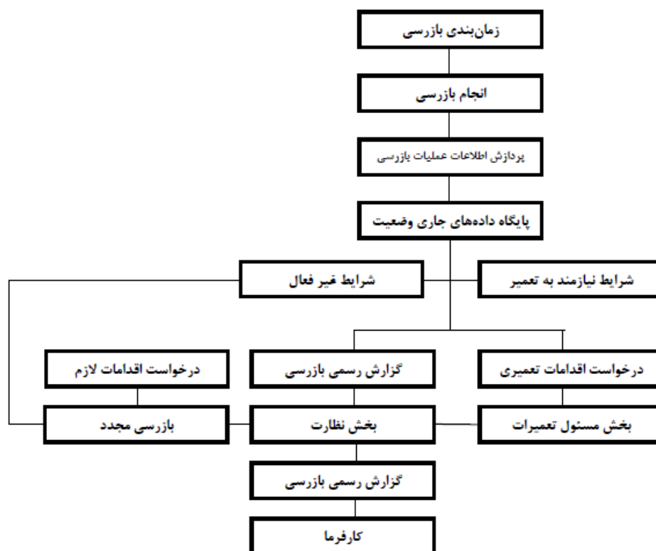
شکل ۱-۳ نمودار فرآیند بازرسی سازه
