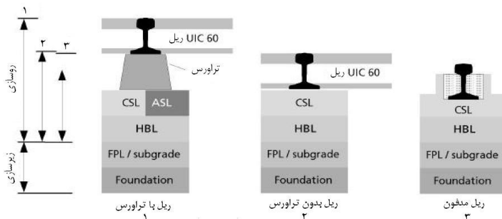
شکل ۲-۱ اشکال مختلف قرارگیری لایه‌های تکیه‌گاهی در خطوط بدون بالاست
