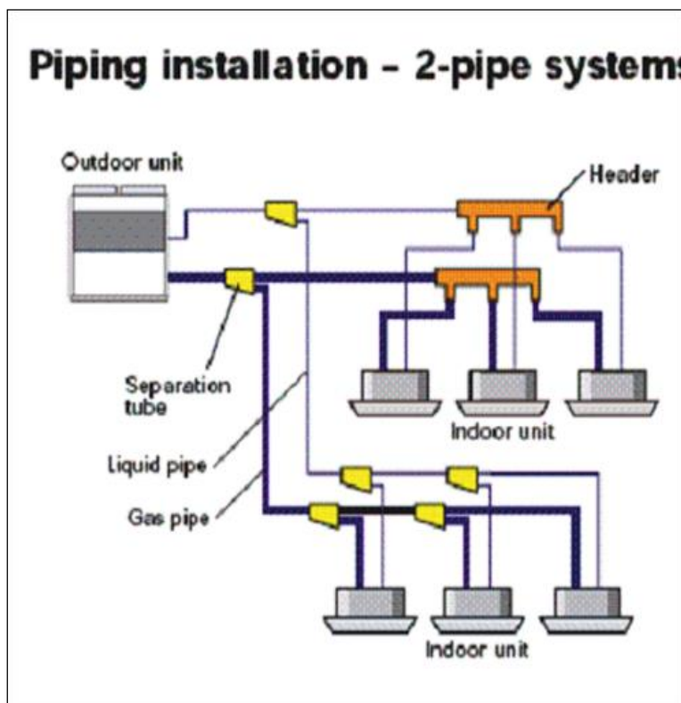
شکل ۲-۲ دیاگرام فلو شماتیک سیستم VRF
