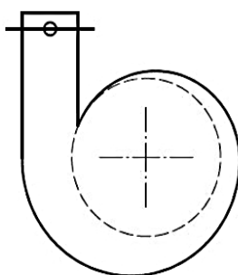
شکل الف-۳ انشعاب فشار عمود بر صفحه مارپیچ یا صفحه خم
