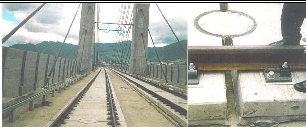
شکل ۲-۲۱ نمونه اجرا شده دال خط شینکانس
