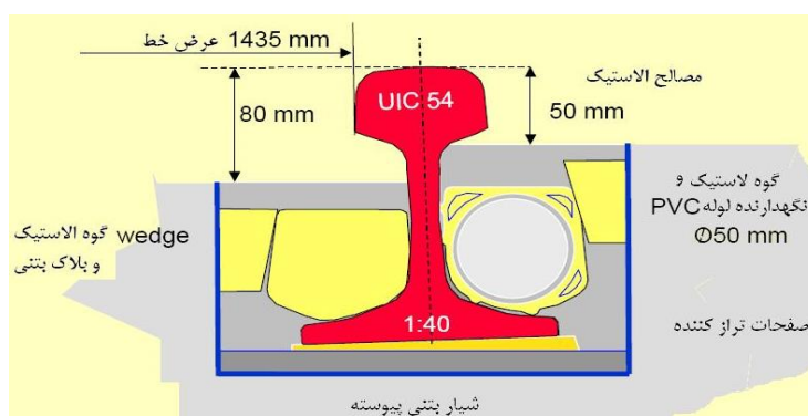
شکل ۲-۲۵ مقطع شیپار طرح ریل مدفون ERC در خطوط معمولی
