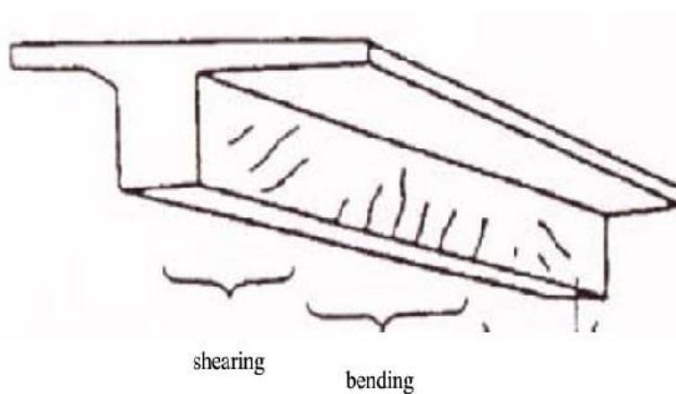
شکل ۵۲ → ترک ناشی از تنش های خمشی و برشی
