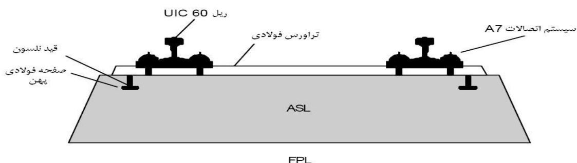
شکل ۲-۱۴ مقطع عرضی طرح ساتو
