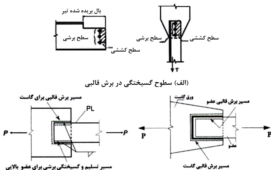
(ب) برخی دیگر از حالت‌های گسیختگی برش قالبی شکل ۱۰-۲-۲- حالت‌های مختلف گسیختگی برشی قالبی
