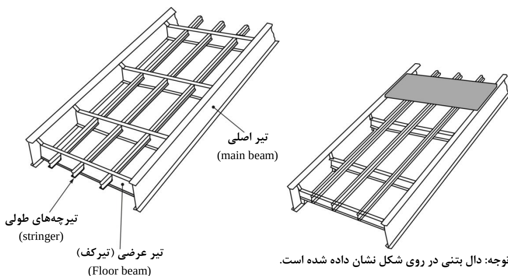
شکل ۲-۶- پلان عرشه چهار عنصری
