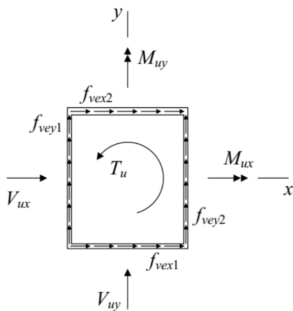
شکل ۸-۲-۳- تنش برشی در مقطع جعبه‌ای تحت ترکیب برش و خمش
