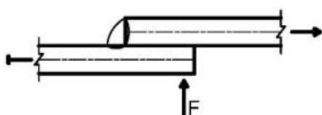
(پ) جوش یک‌طرفه مقید و مجاز
