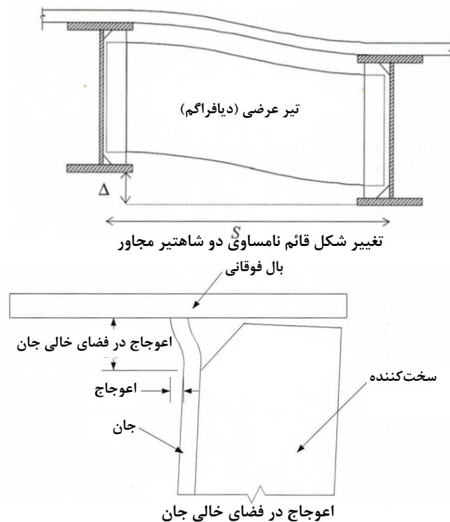
شکل ۱۱-۴- خستگی اعوجاجی
