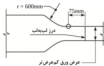
(پ) تبدیل با کمان r = 600 \text{ mm}
