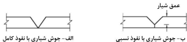
شکل ۹-۱-۱- جوش شیاری
