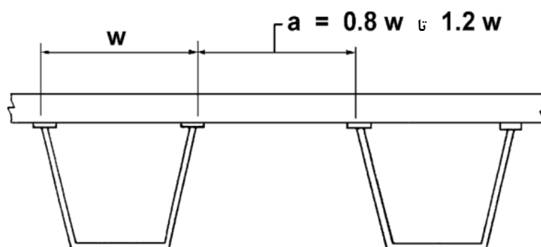
شکل ۶-۱-۱-الف- فواصل تیرورق‌های جعبه‌ای
