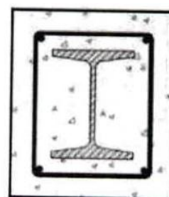
(الف) عضو محوری مختلط محاط در بتن (روکش بتنی و هسته‌ی فولادی)
