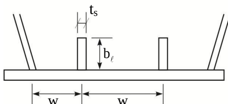
شکل ۶-۳-۲- سخت‌کننده‌های طولی و فواصل آنها
