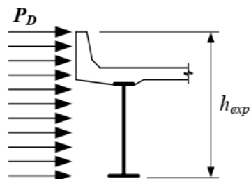
شکل ۲۸- نیروی باد
