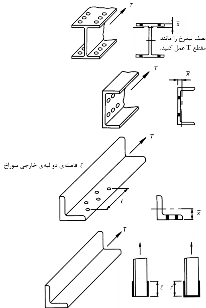
شکل ۳-۴- تعیین \bar{x} و \ell در محاسبه‌ی تاخیر برشی و ضریب کاهش U
