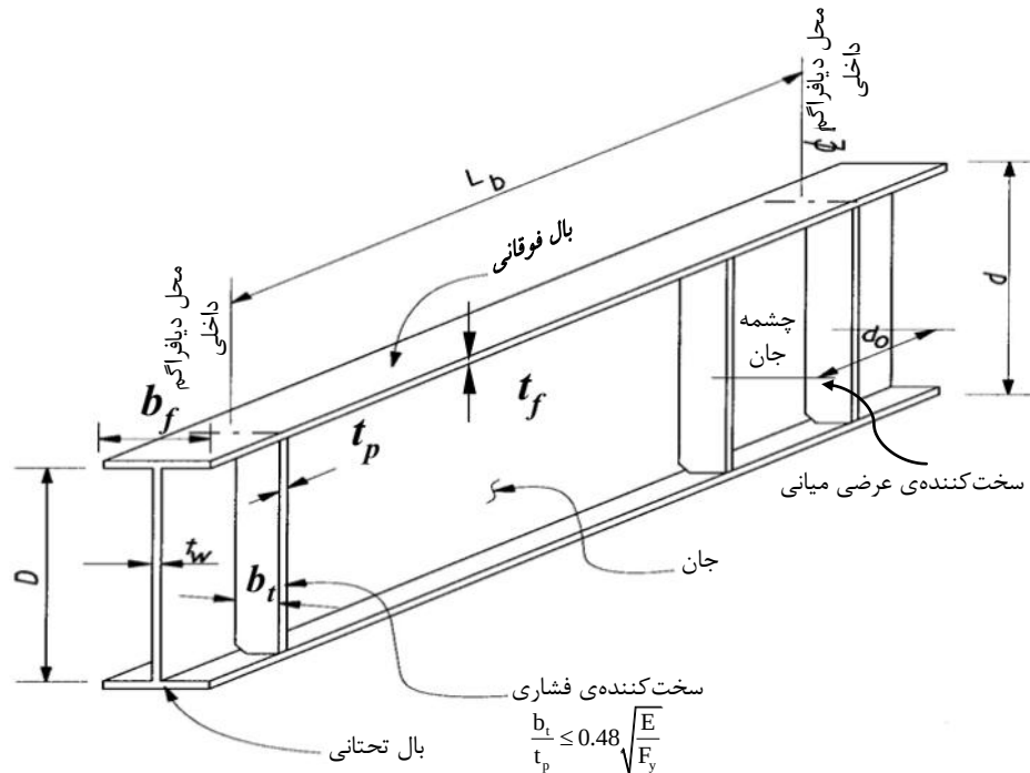
شکل ۱-۴-۱- تناسبات ابعادی تیرورق
